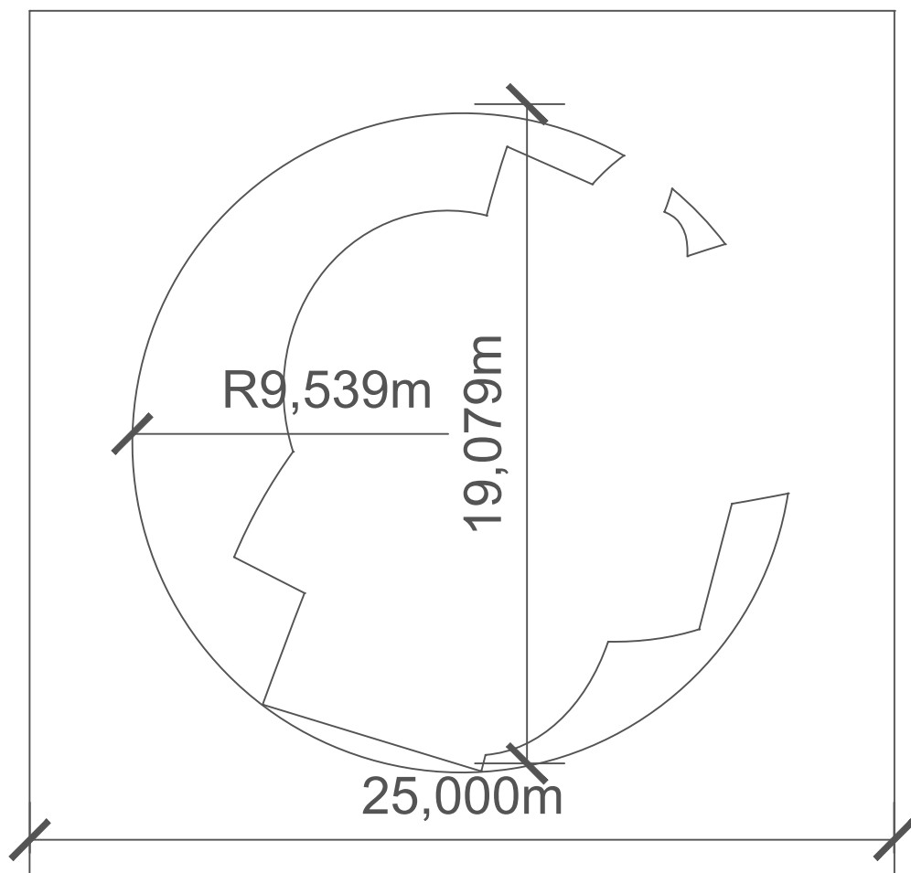
planta 1:200
