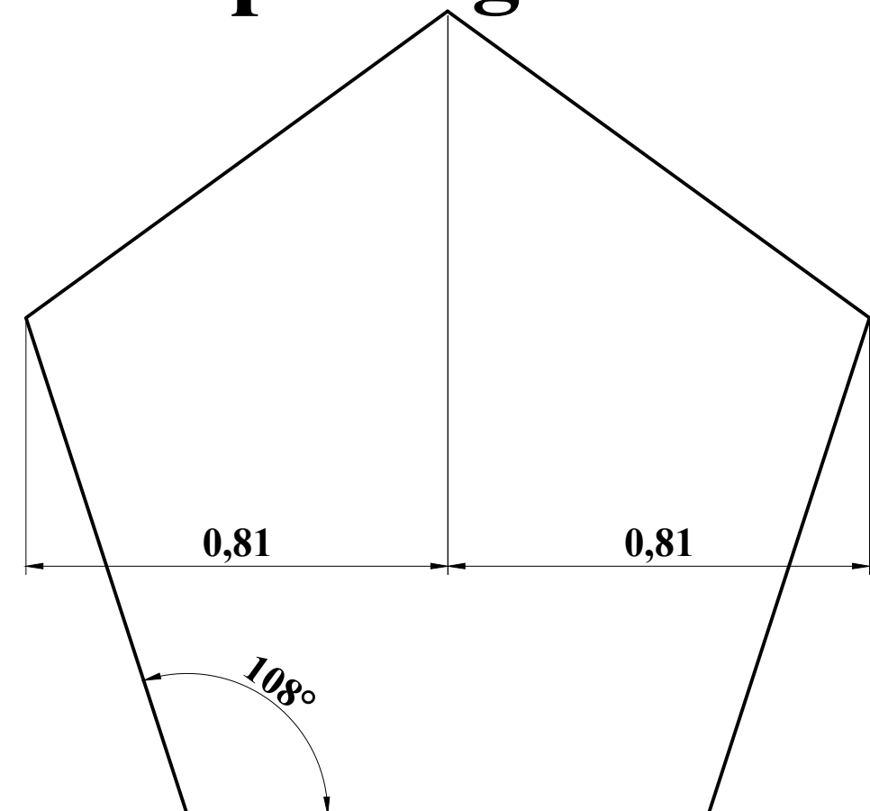
pentágono
