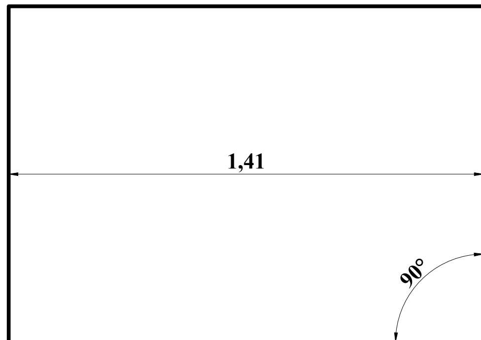
retângulo aureo
