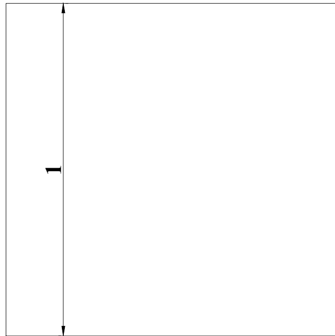
quadrado
