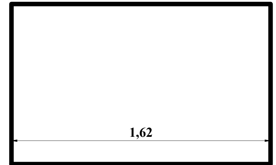
retângulo r2
