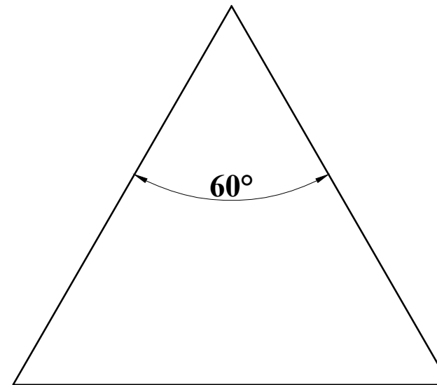
triângulo
