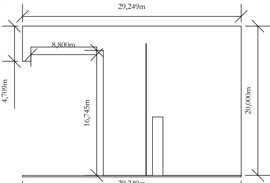
Corte longitudinal
