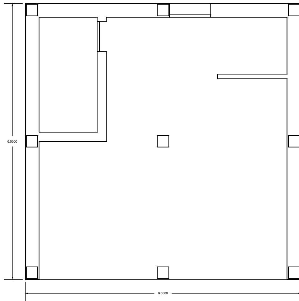
Planta Baixa
