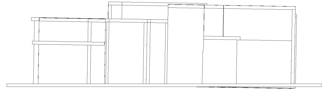
ALÇADO NORTE 1:150
