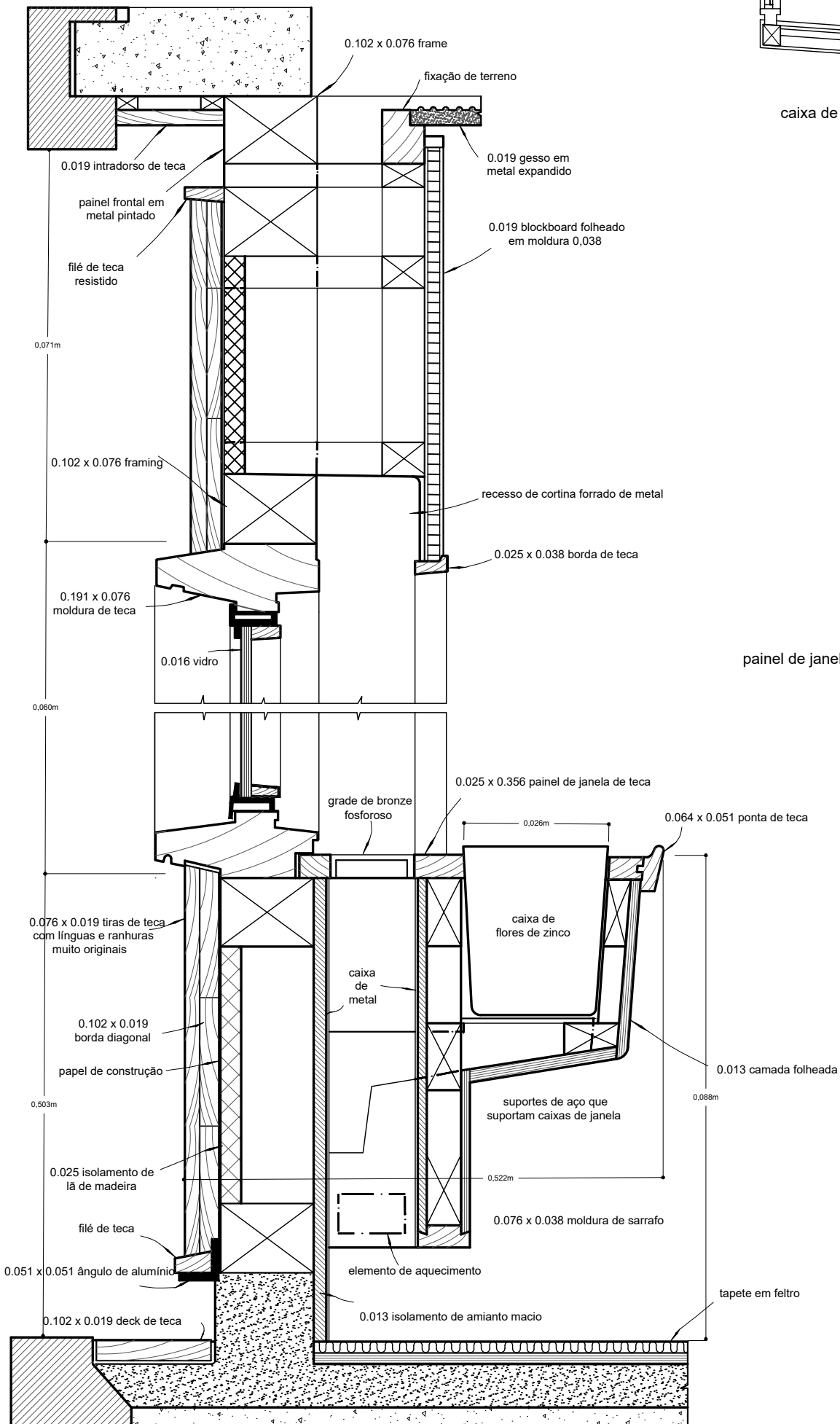
SECÇÃO ATRAVÉS DA JANELA NA BAIJA DO RESTAURANTE ESCALA 1- 6
