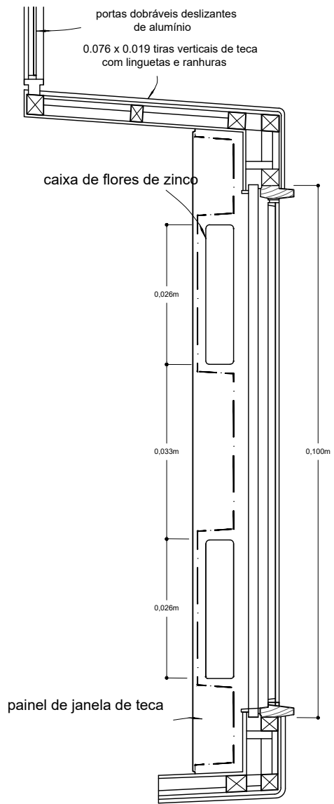
PLANO DE PARTE DA BAIJA DO RESTAURANT ESCALA 1-32
