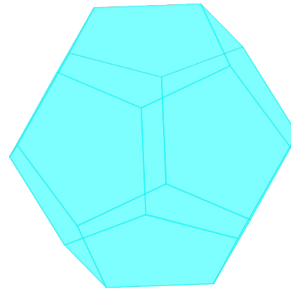
DODECAEDRO
