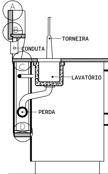
CORTE VERTICAL PELO LAVATÓRIO
