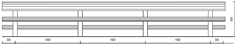
ELEVATION
