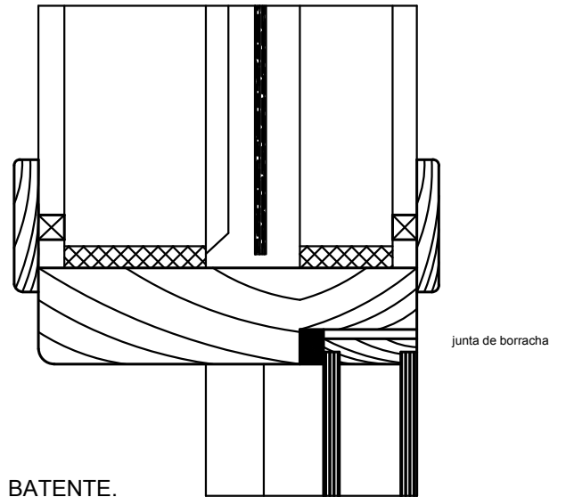
BATENTE.
