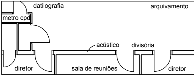
PLANO DE LAYOUT COM DIVISÕES ACÚSTICAS.
