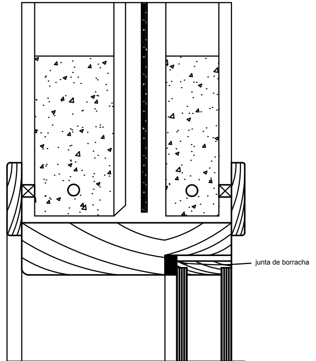
CABEÇA.
