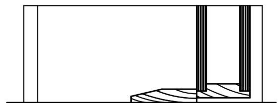
DETALHES DA PORTA.
