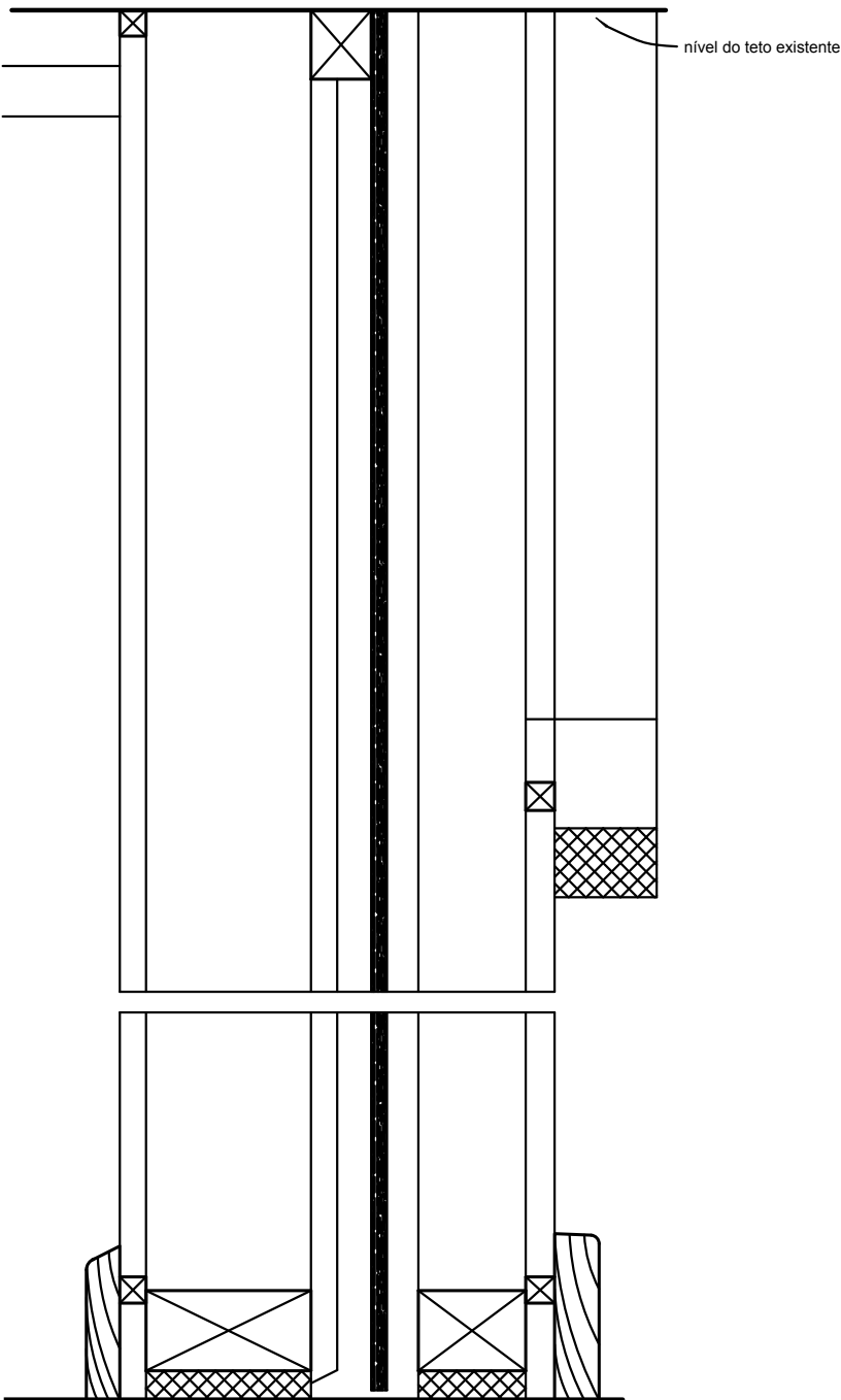
SECÇÃO ATRAVÉS DA PARTIÇÃO.
