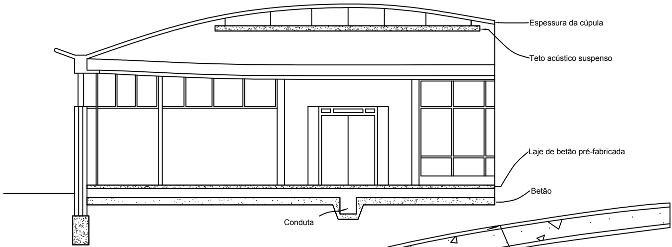
PARTE DO CORTE SOBRE "ASSEMBLY HALL"
