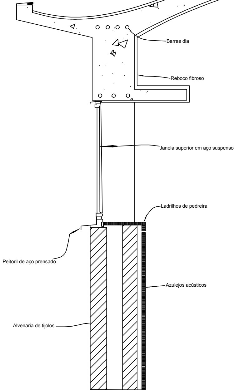
DETALHE DA PAREDE EXTERNA E BEIRADOS. Escala: 1/16
