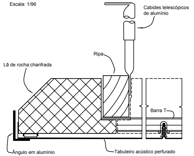
CORTE A-A. ESCALA 1/4
