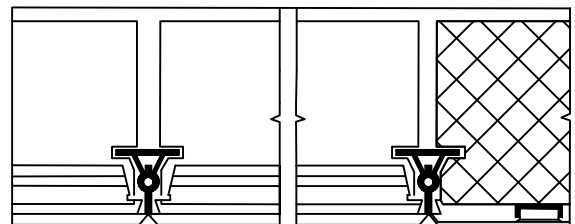
CORTE B-B. ESCALA 1/4
