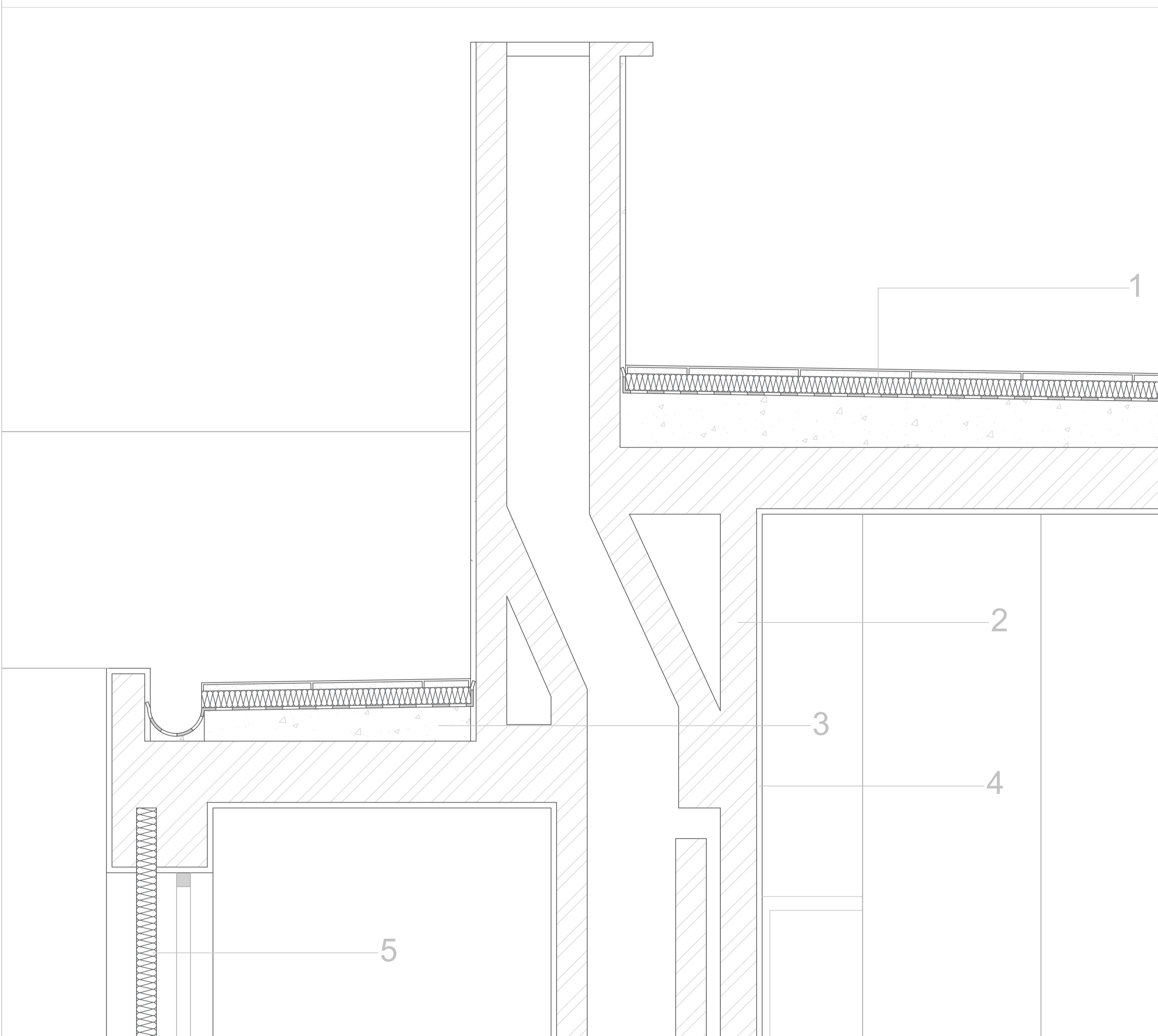
PORMENOR - CHAMINÉ ESCALA 1:10
