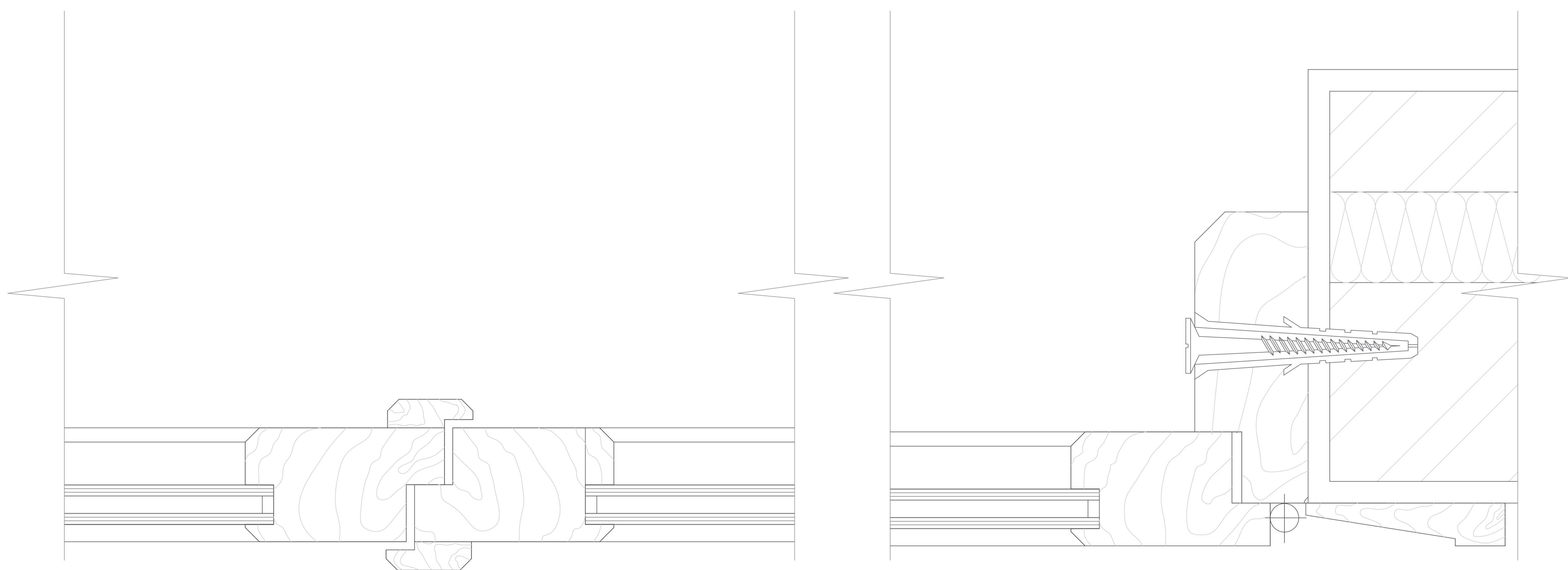
PORMENOR - CAIXILHARIA ESCALA 1:2
