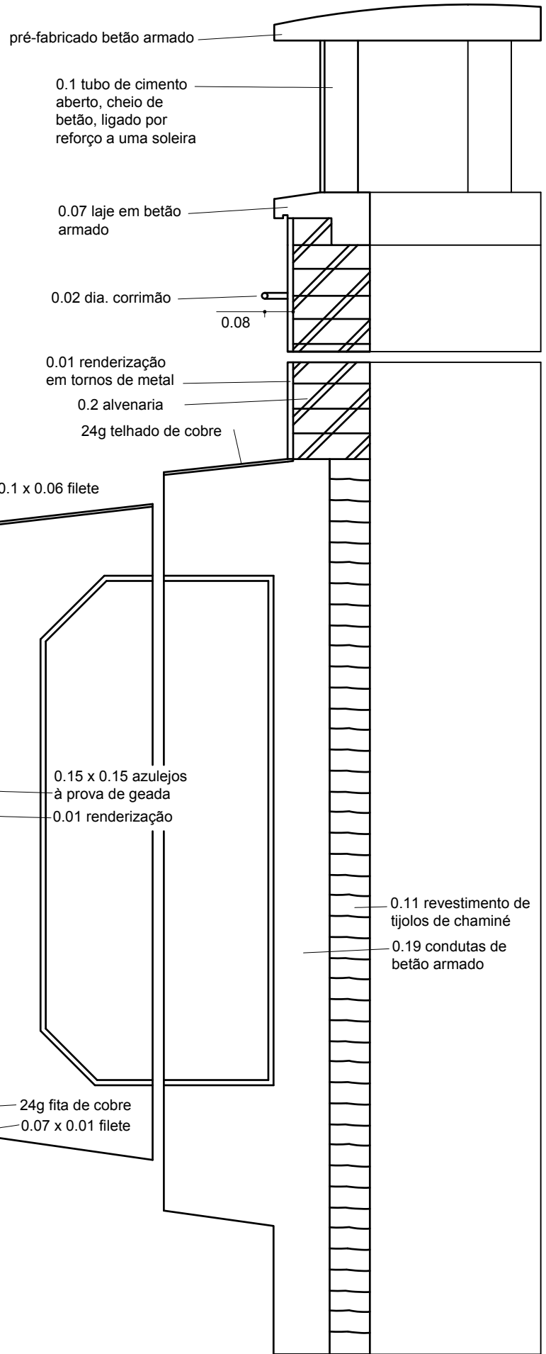
SECÇÃO DO TANQUE. escala 1:16
