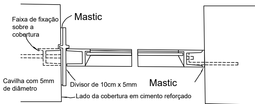
Detalhe de A. Escala 1/4
