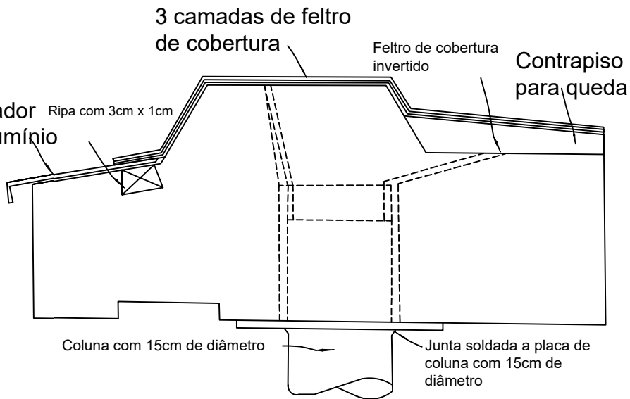
Detalhe dos Beirais Escala 1/4
