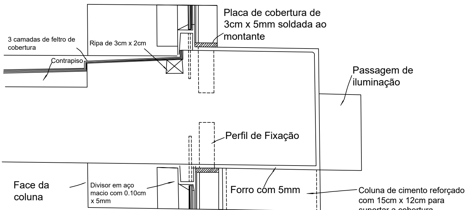
Detalhe de B. Escala 1/4
