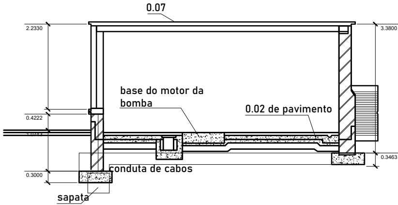
SECÇÃO A-A escala 1/96
