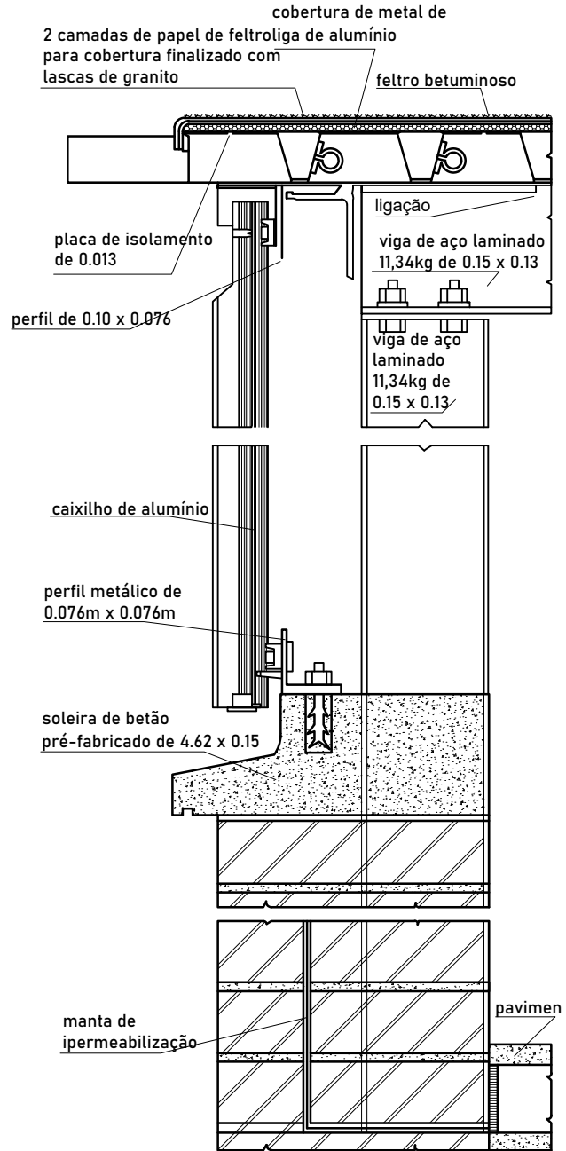
CORTE PELA JANELA escala 1/8
