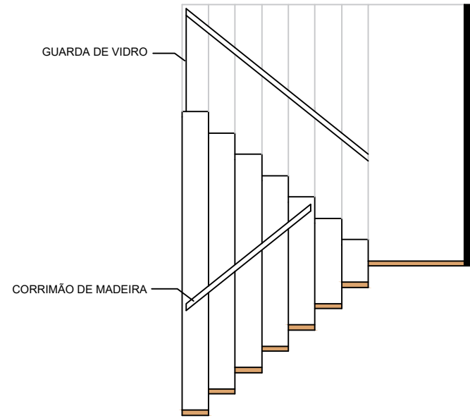
CORTE TRANSVERSAL
