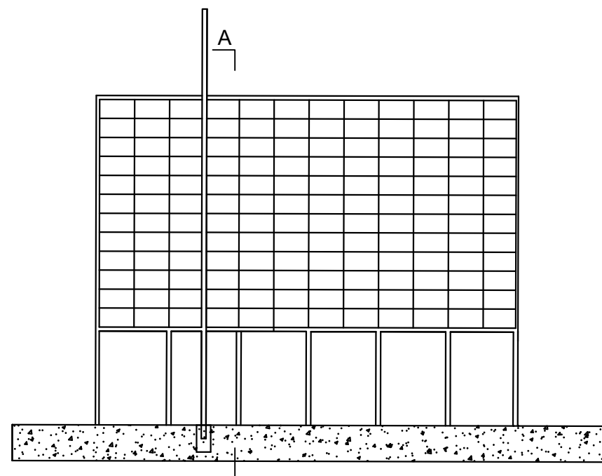
Elevação 1:50
