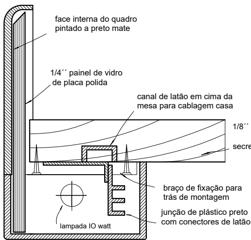
SECÇÃO A - A escalas 1/2 full size
