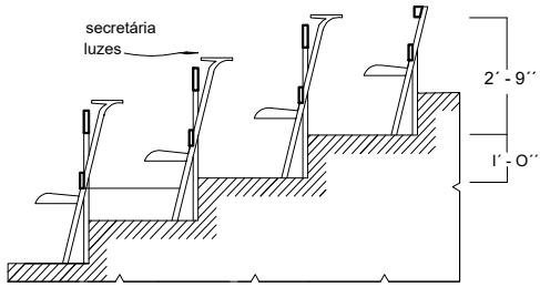
SECÇÃO escala 1/4" - 1'-0"
