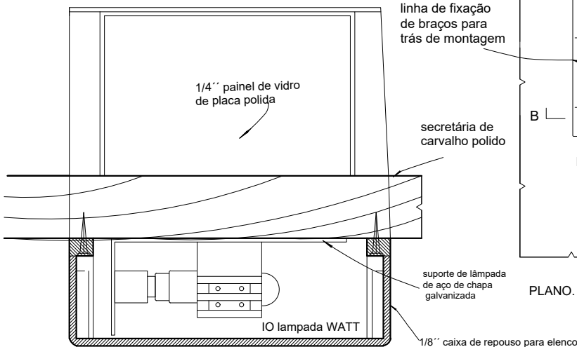
SECÇÃO A - A escalas 1/2 full size
