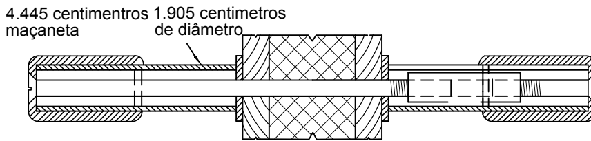
seção e plano a mostrar as maçanetas
