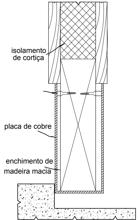
seção vertical escala 1:2
