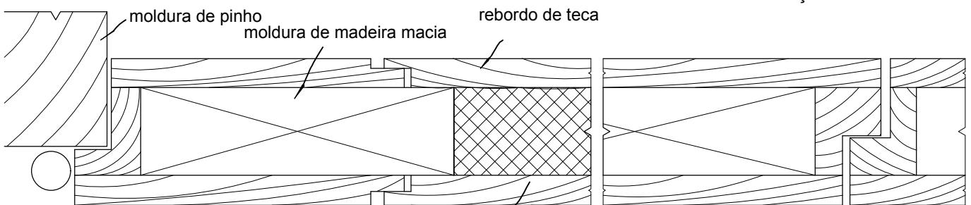
seção vertical escala 1:2
