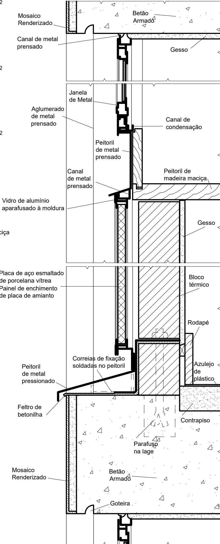
Corte 1/64
