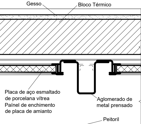
Planta 1/64
