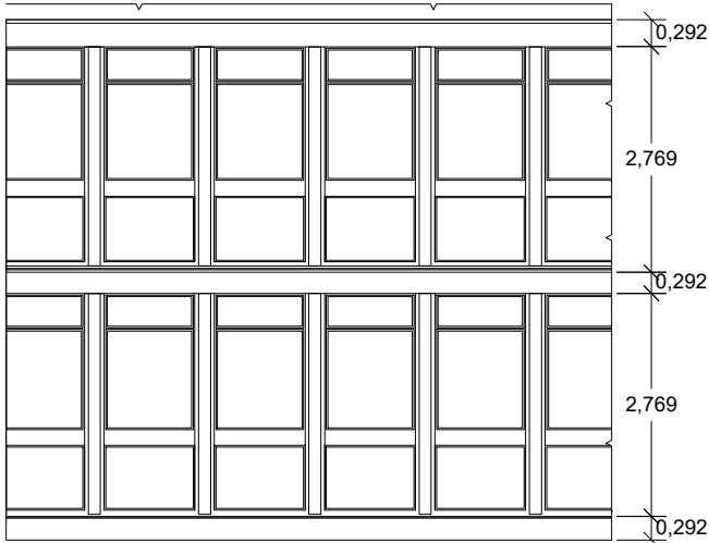
Alçado 1/100
