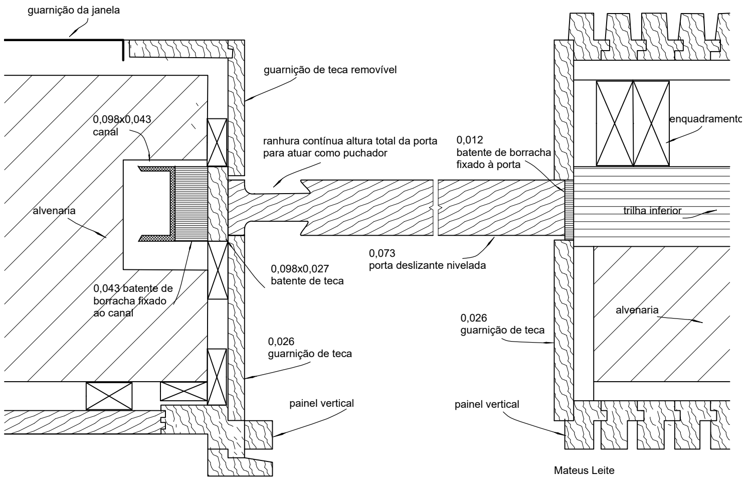
Planta B-B Escala 1/5
