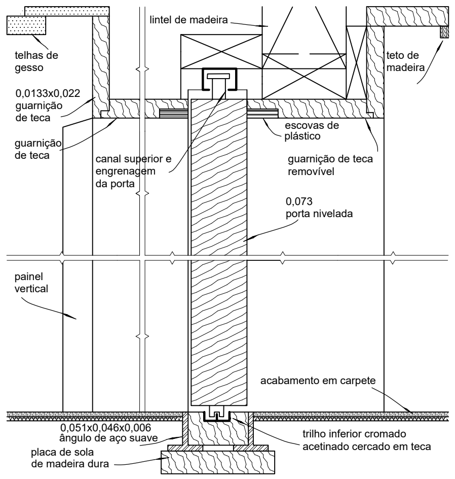
seção A-A escala 1/5
