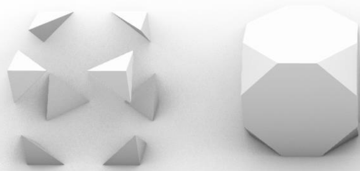
Cubo Truncado a 1/3 da aresta
