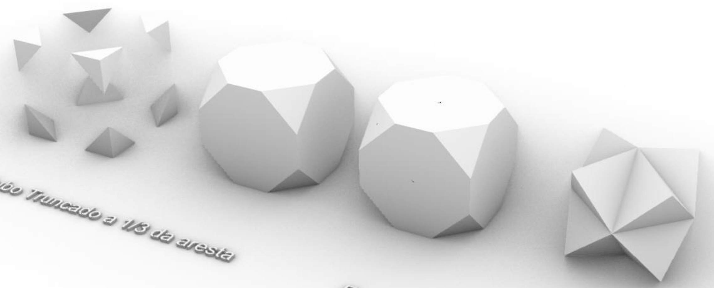
Dual do Cubo Truncado
