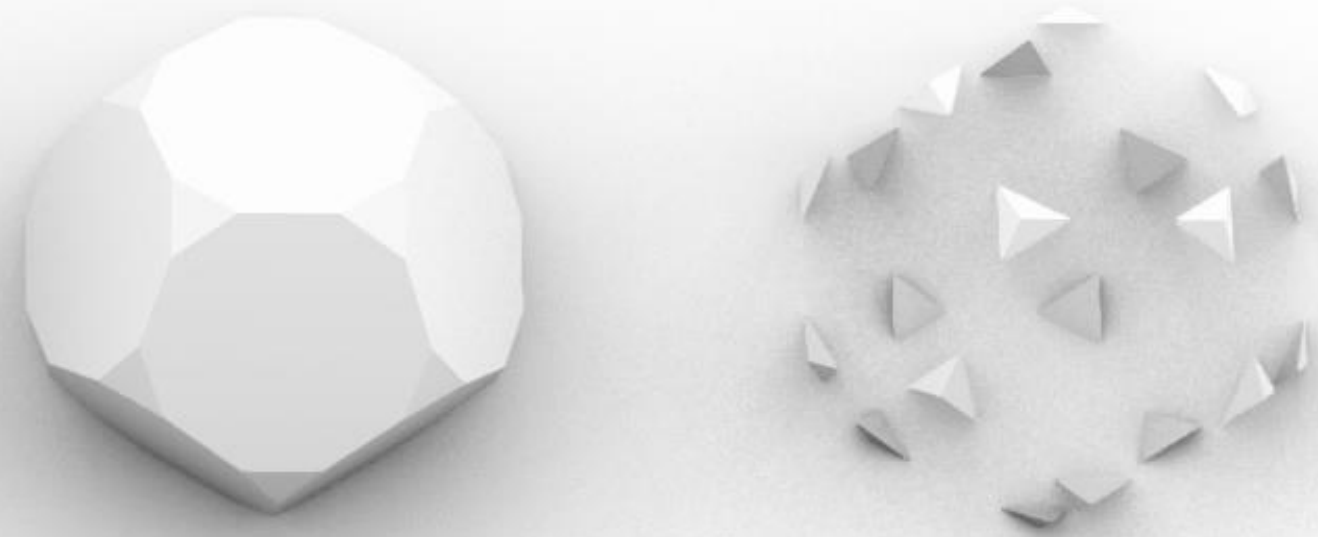
Dodecaedro Truncado
