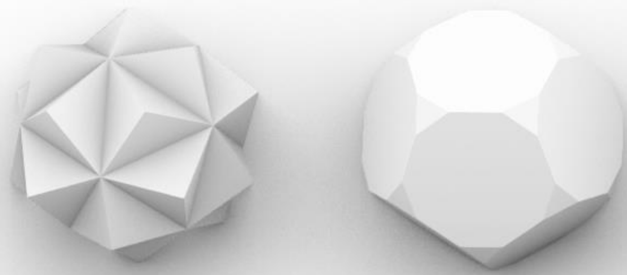
Dodecaedro Truncado a 1/4 de aresta
