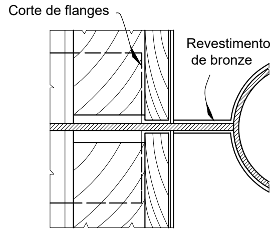
Plano "B", Escala 1/4, tamanho real
