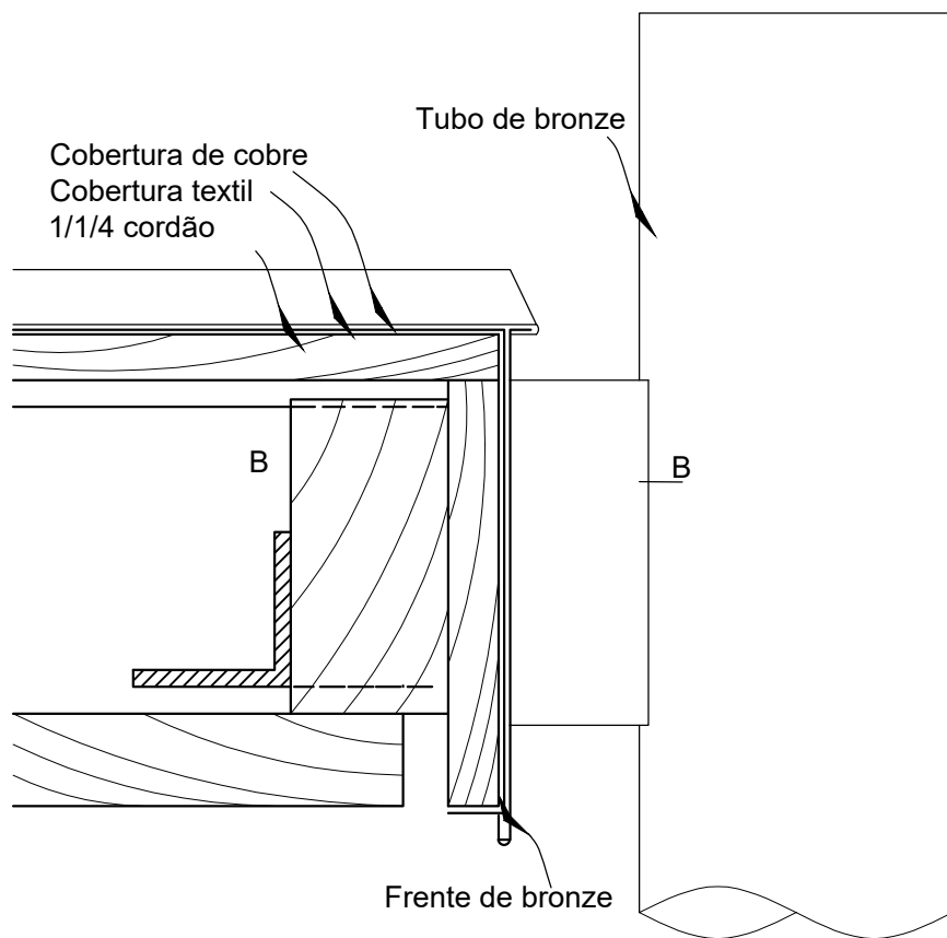
Detalhe "A", escala 1/4, tamanho real
