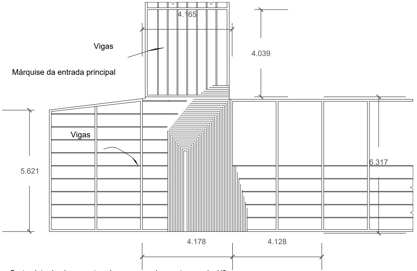
Corte visto de cima mostrando um enquadramento, escala 1/8
