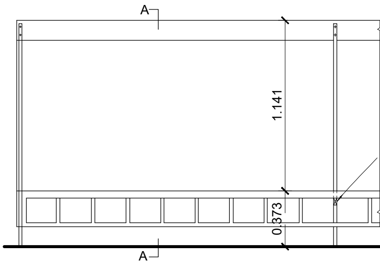
ELEVAÇÃO escala 1/25
