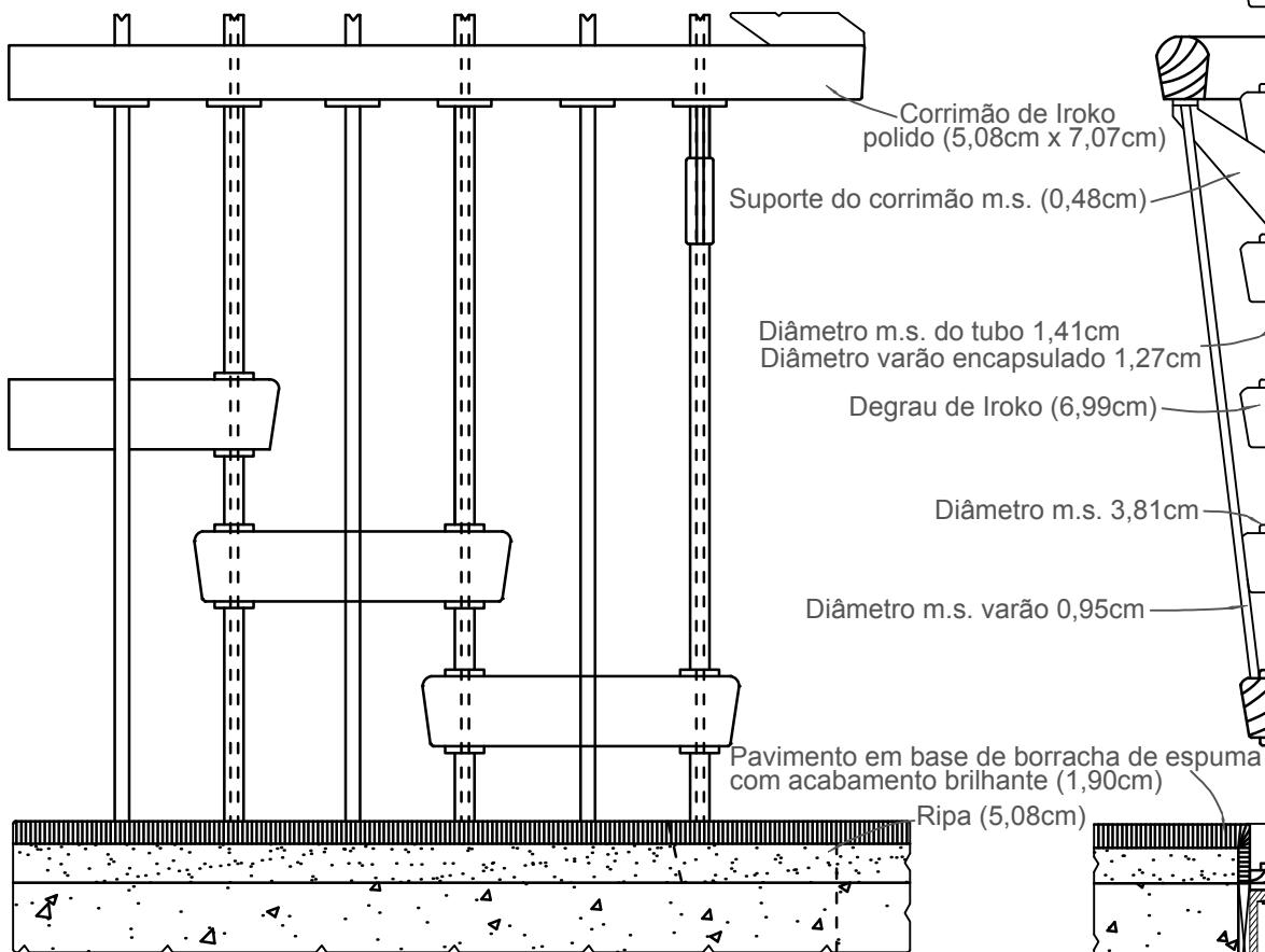
ALÇADO Escala 1/8
