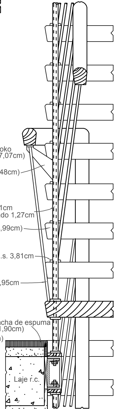
CORTE A-A Escala 1/8
