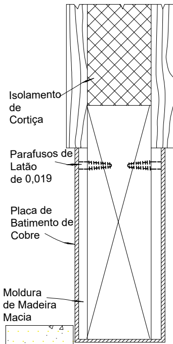
Secção Vertical
