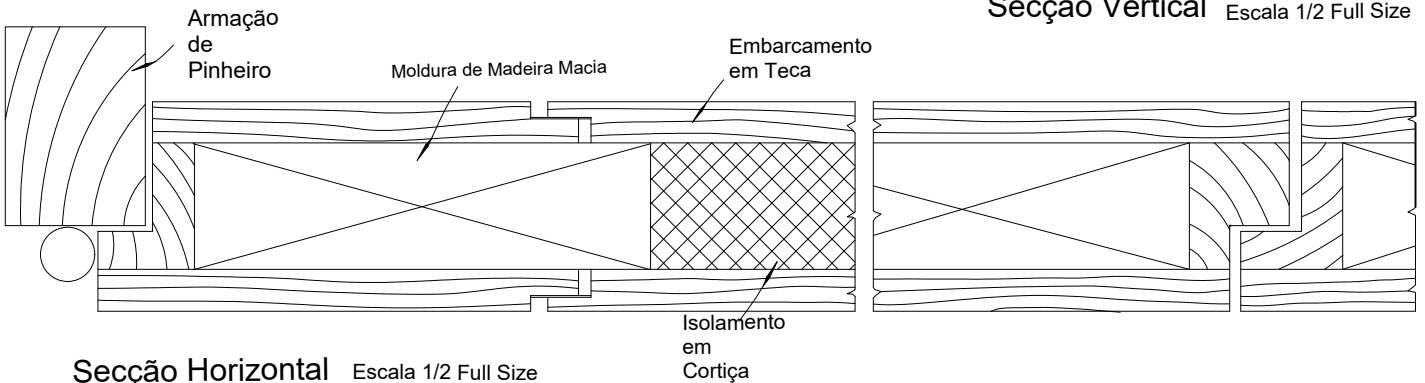
Secção Vertical
