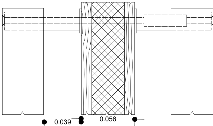
Alçado
