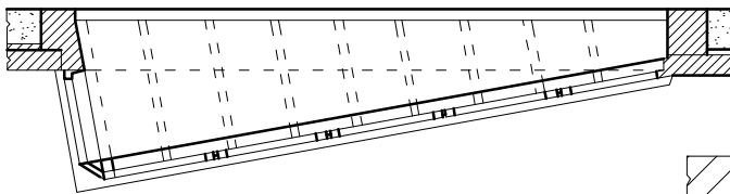
ALÇADO E PLANTA Escala 1/50
