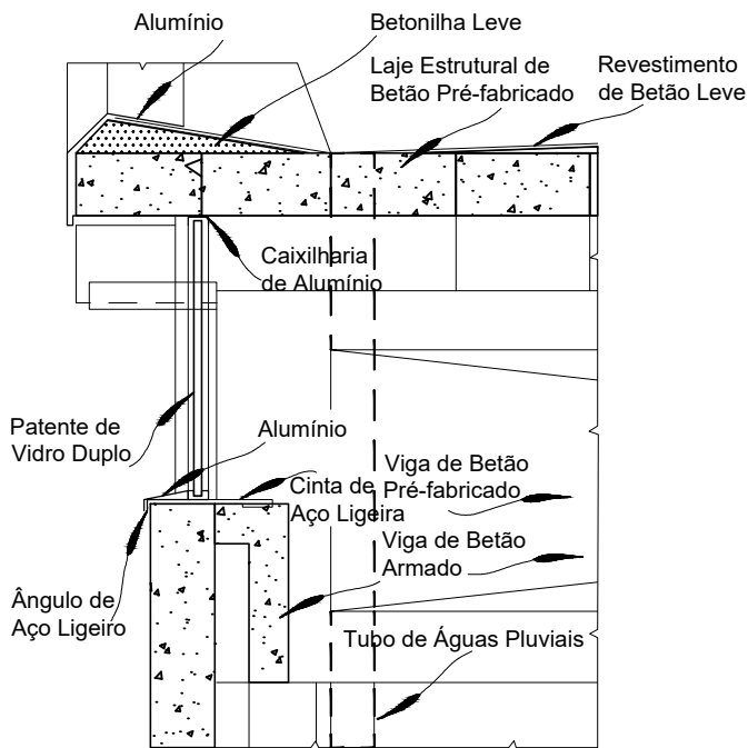
Corte em C - C Escala \frac{1}{30}
