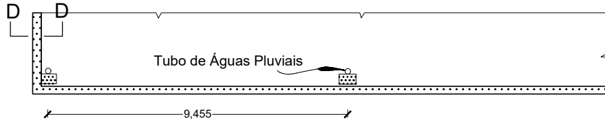
Planta em A - A Escala \frac{1}{160}
