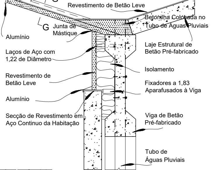
Detalhe de G - G
