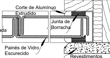
Detalhe de F Escala \frac{1}{3}
