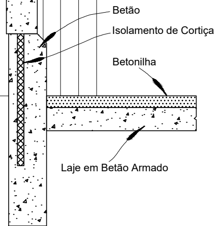
Corte de D - D Escala \frac{1}{30}
