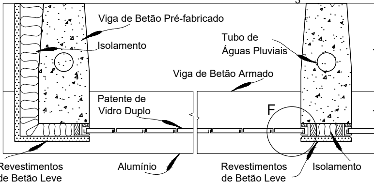
Planta em B - B Escala \frac{1}{30}
