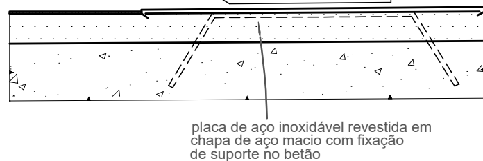
DETALHE C 1:8
