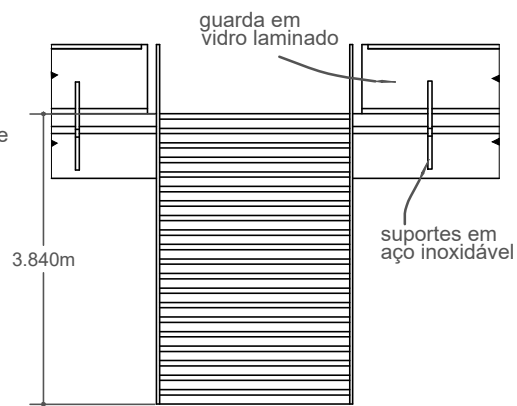
ALÇADO FRONTAL 1:100
