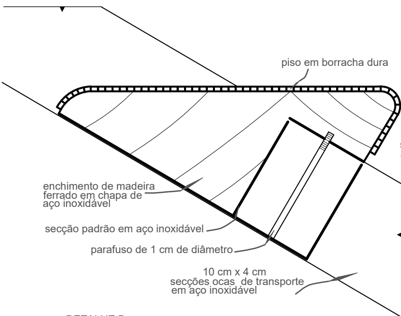
DETALHE B 1:4
