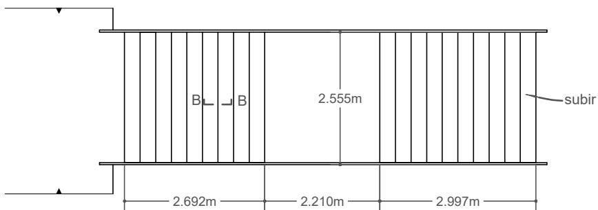
PLANTA 1:100
