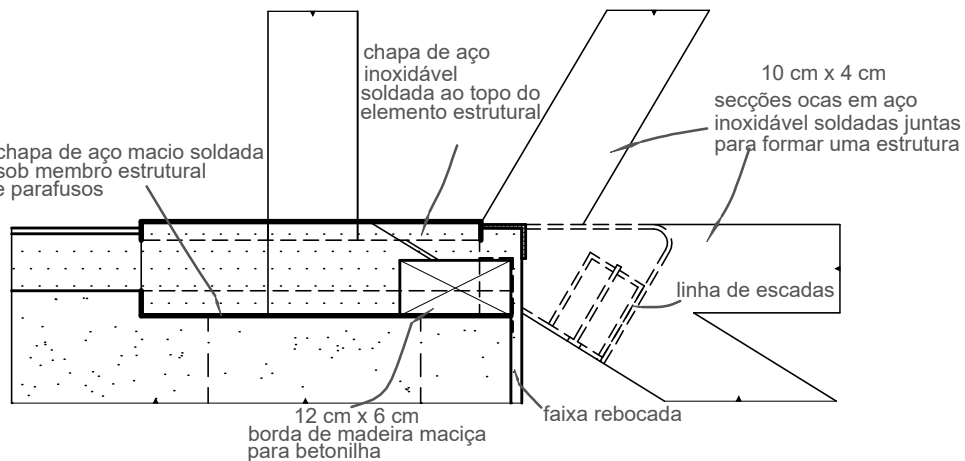
DETALHE A 1:8
