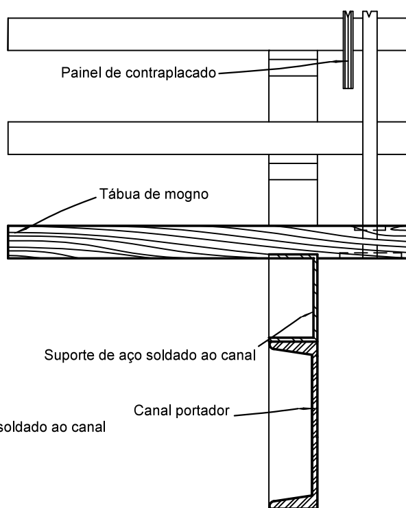
Escala 1/2 Detalhe Corrimão
