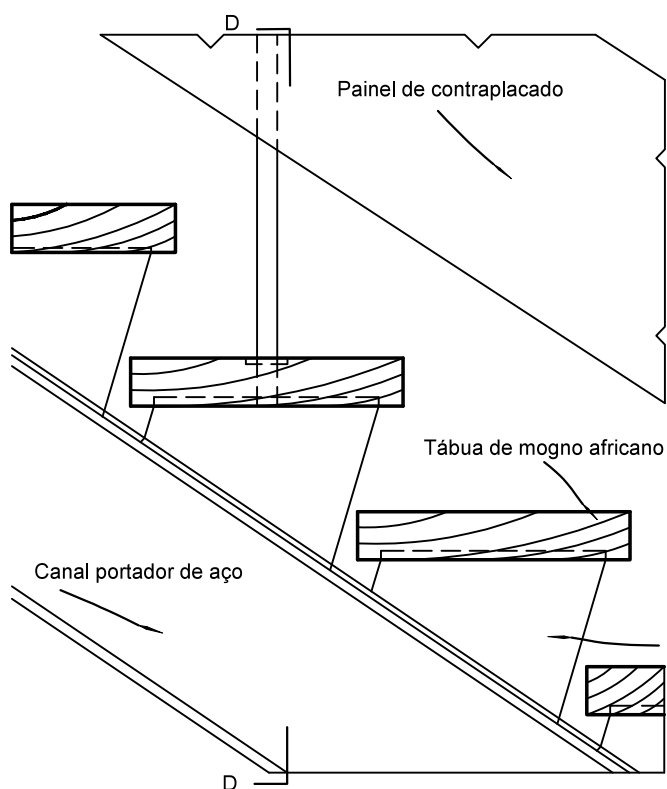
Escala 1/8 Corte C
