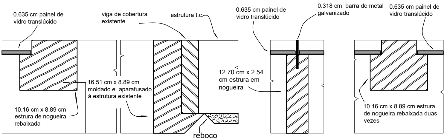
CORTE B - B. escala 1/4
