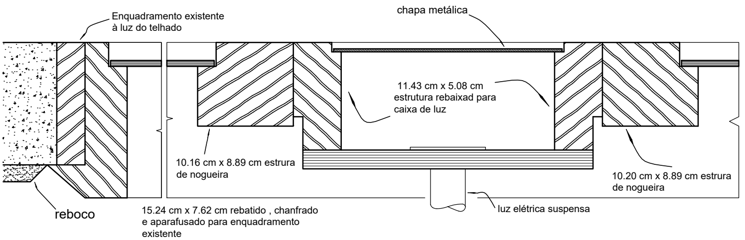
CORTE A - A. escala 1/4
