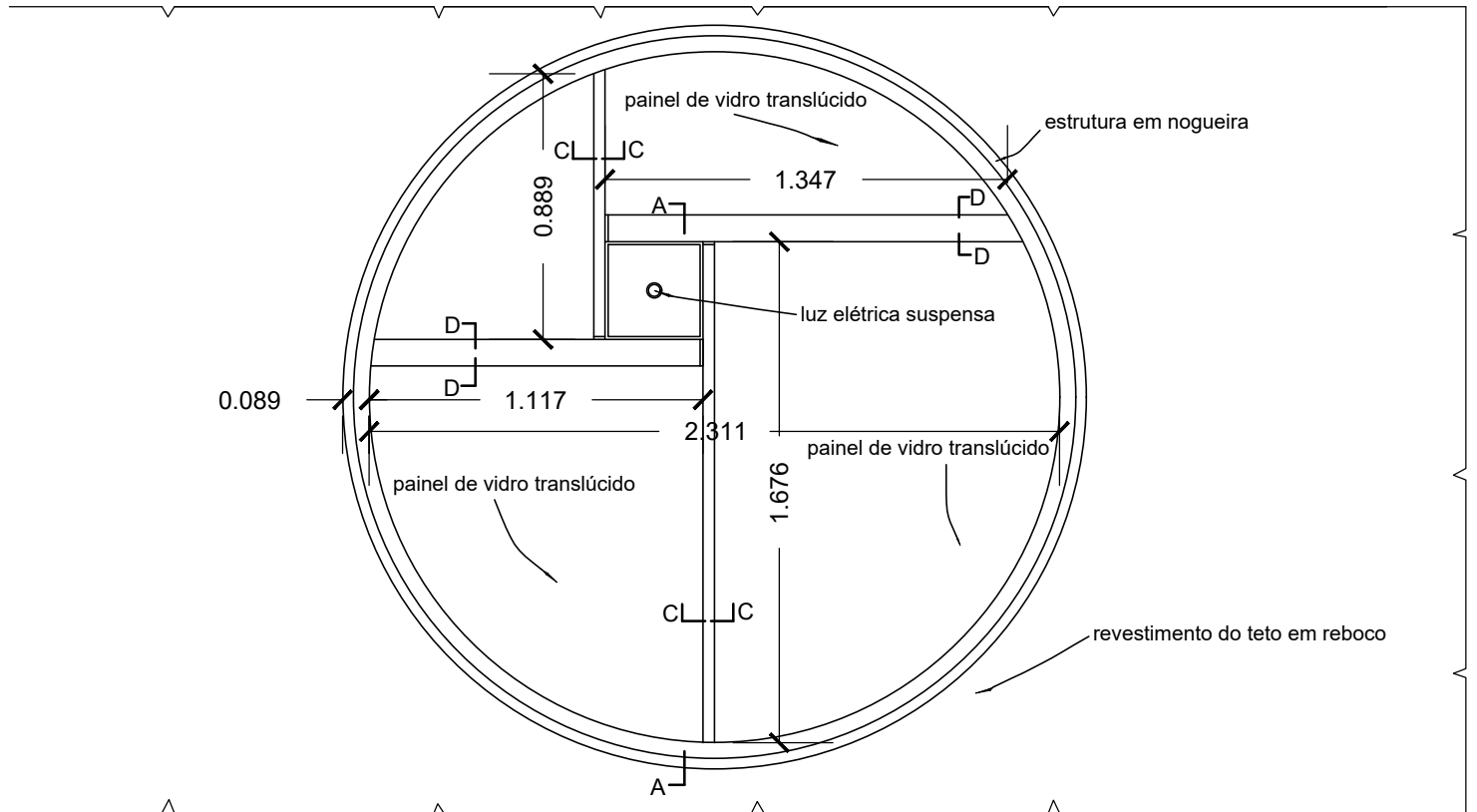
PLANO VISTO DE BAIXO escala 1/25
