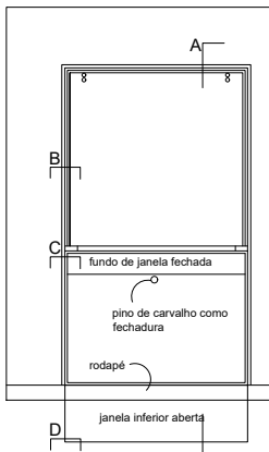
elevação interna duma janela típica esc. 1/24
