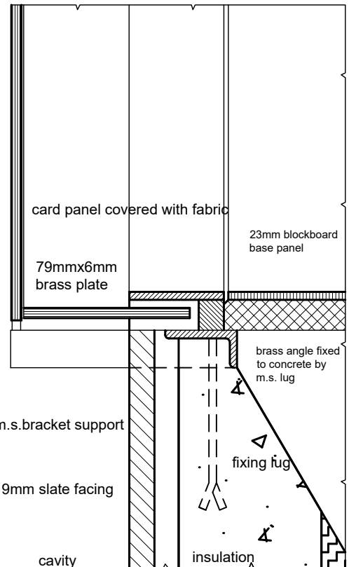
SECTION A-A scale 1:4
