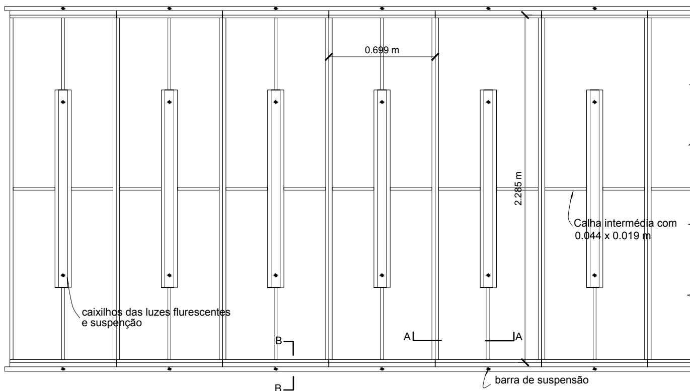
Planta de teto suspenso. escala 1/25
