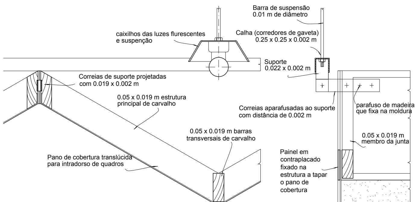
Corte A-A. escala 1/4 tamanho real
