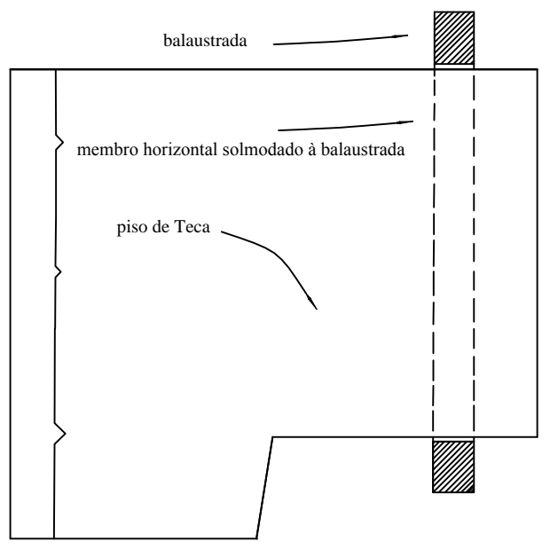
PARTE DO PLANO DE CORTE esc. 1/5
