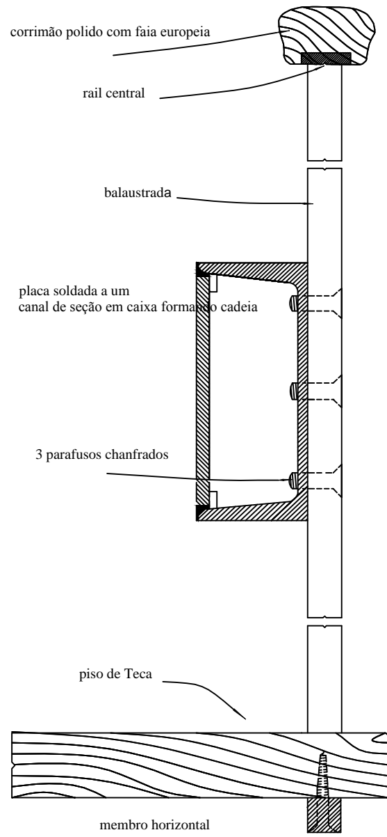
Secção B-B. esc. 1/5
