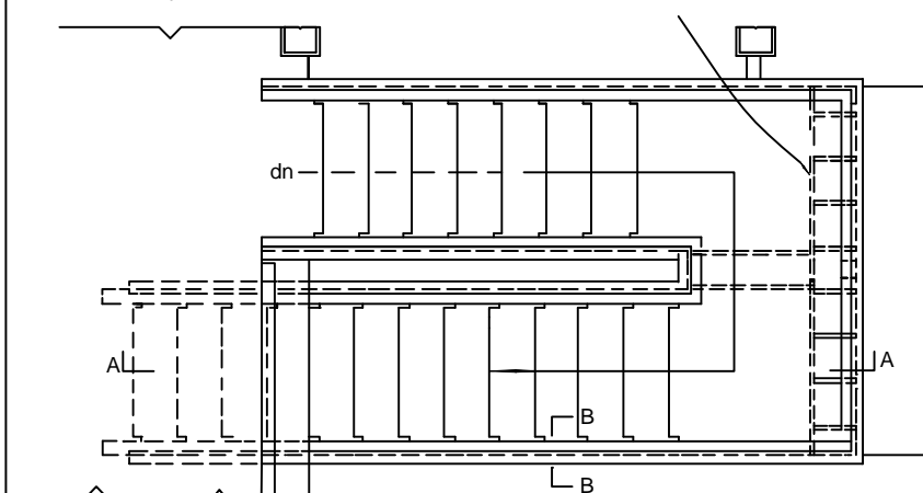
PLANTA esc. 1/50
