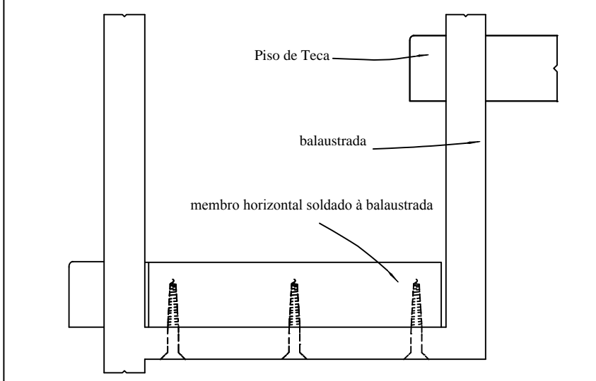
ELEVAÇÃO FINAL DE PISO
