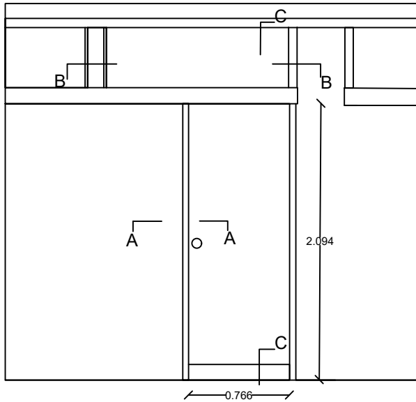
Alçado escala 1/40
