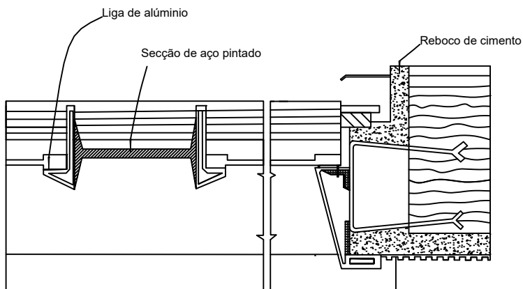
Secção B escala 1/4
