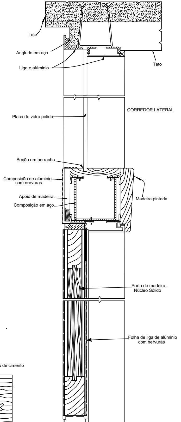
Secção C escala 1/4
