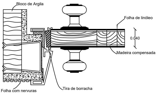
Secção A escala 1/4
