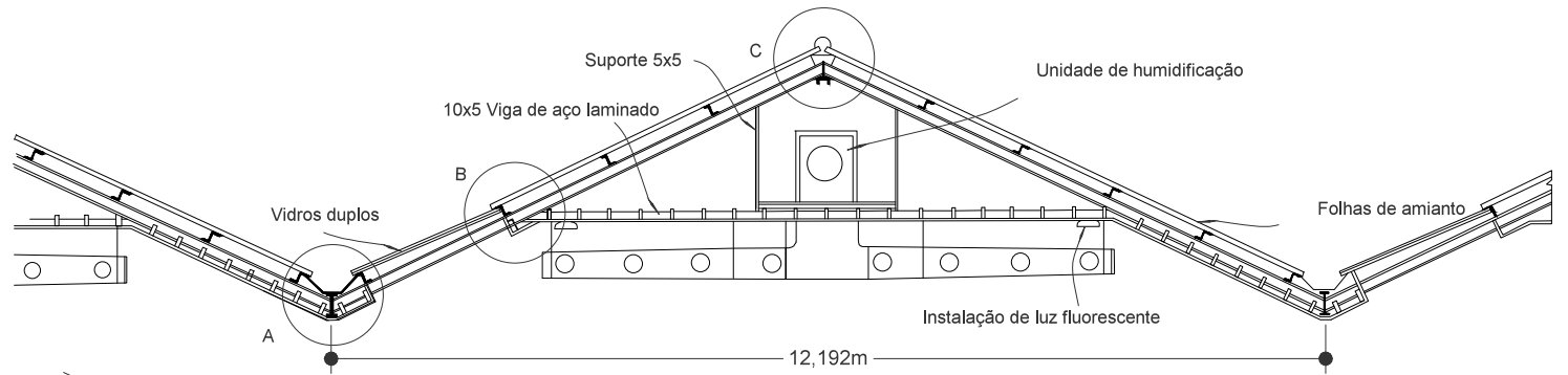
CORTE. Escala 1/96
