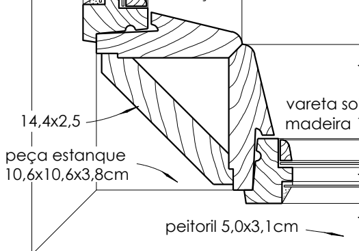
CORTE HORIZONTAL - JANELA. escala : 1/4
