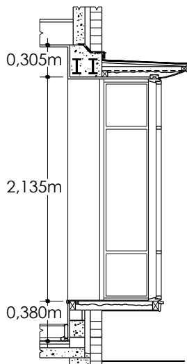
corte
