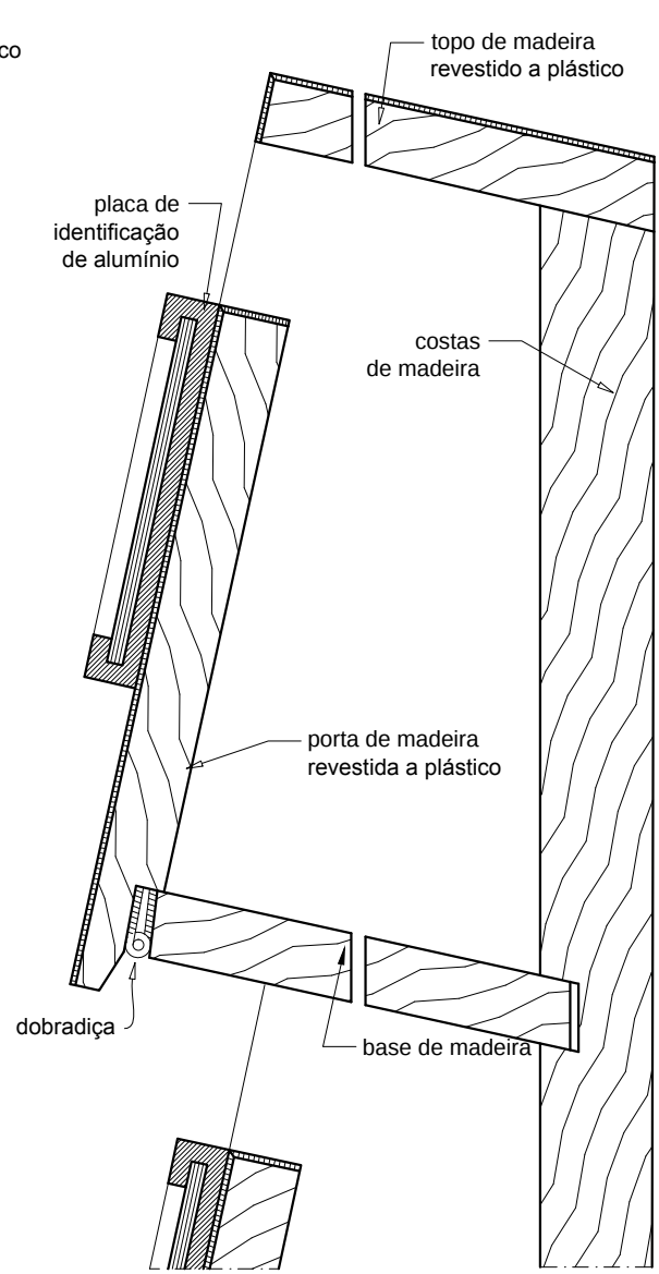
CORTE C-C. escala real
